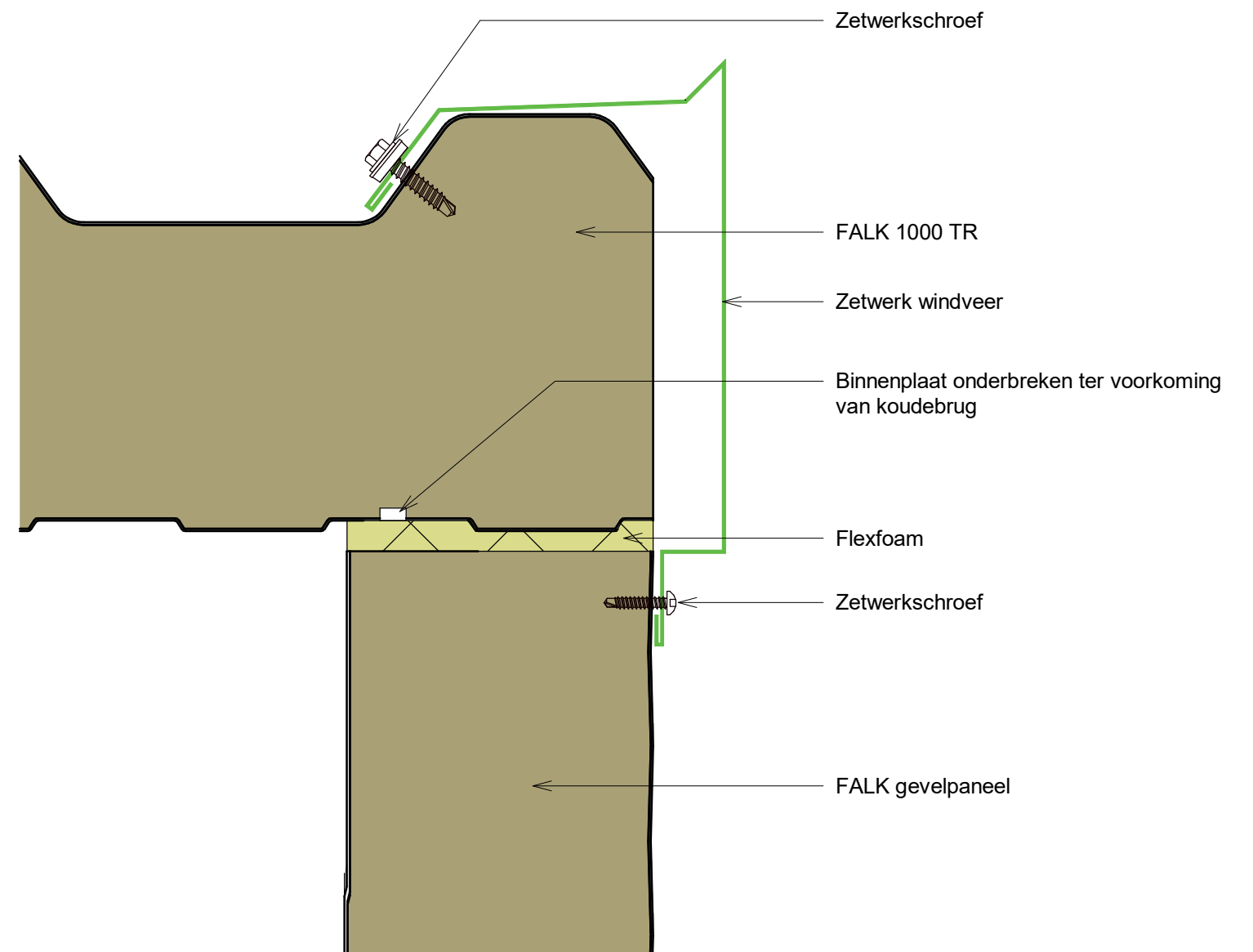
11 DETAIL windveer 1 : 2
