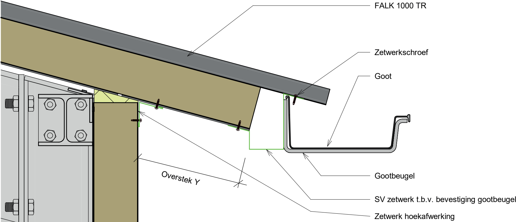
Overstek Y bij gootzijde:
