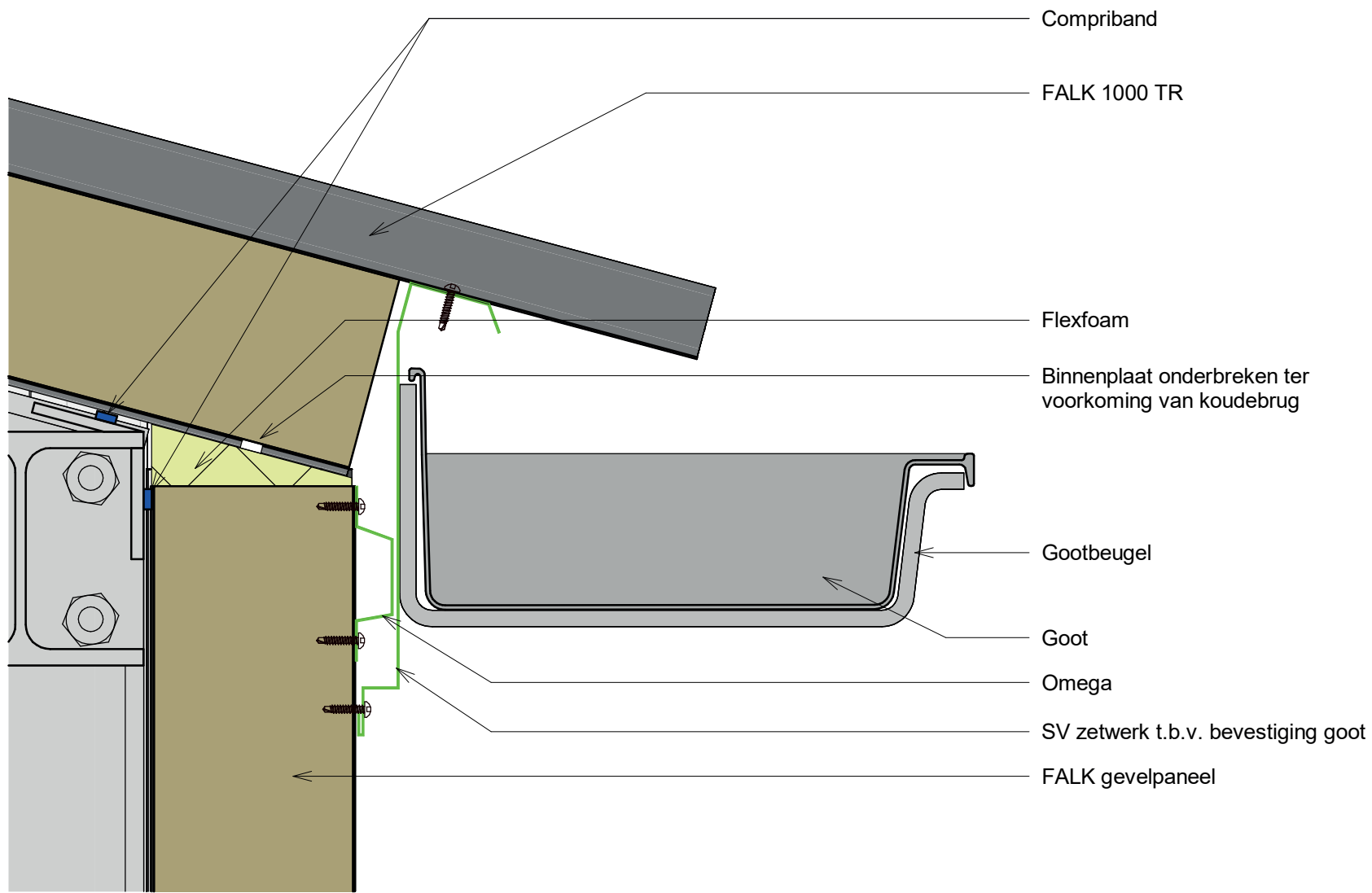
10 DETAIL goot gevelbevestiging 1 : 3
