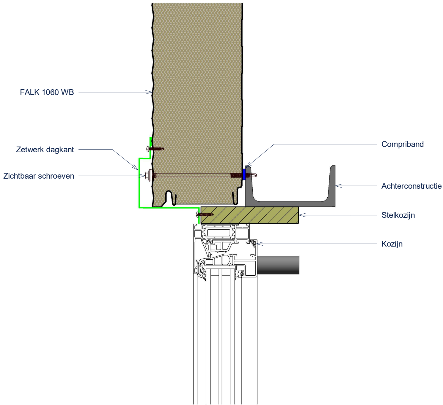
03-Detail dagkant kozijn 1 : 3
