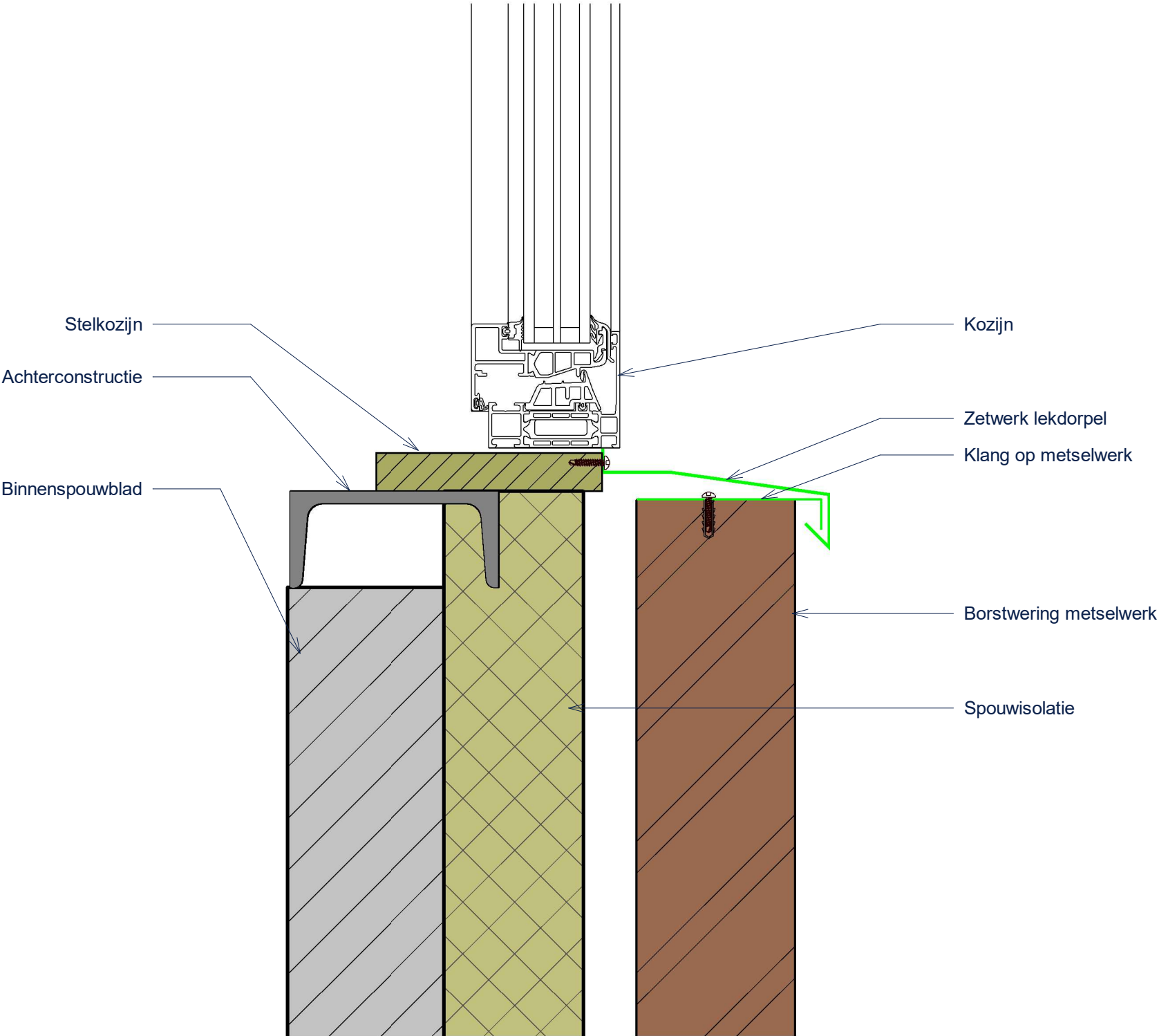
01-Detail onderaansluiting 1 : 3
