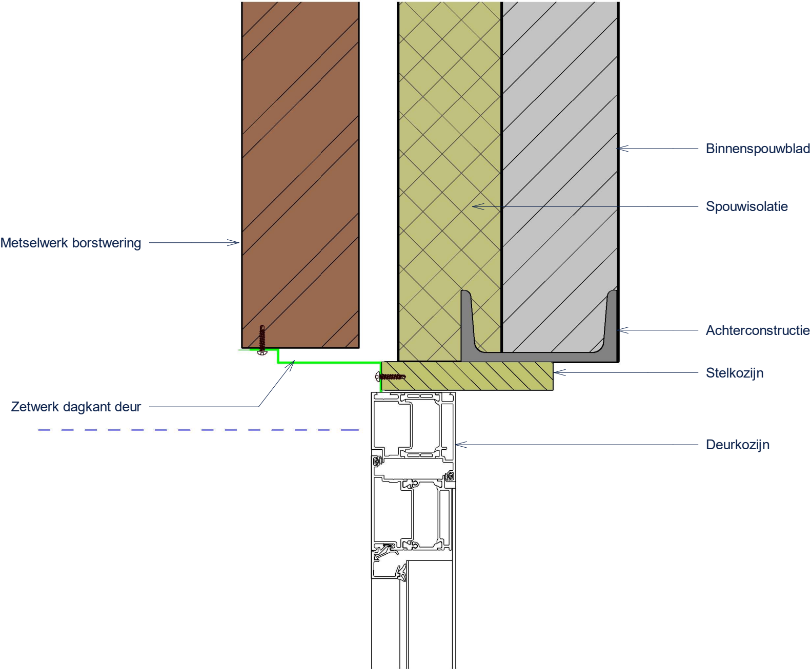
04-Detail borstwering 1 : 3
